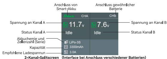
2-Kanal-Splitscreen (Interface bei Anschluss verschiedener Batterien)
